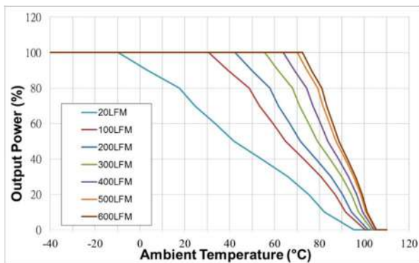
图 3: 环境温度 VS 输出效率额降曲线
