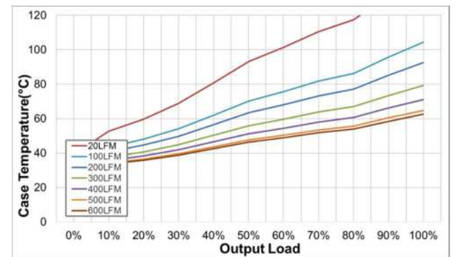
图 4: 工作亮温 VS 输出负载(满载)
