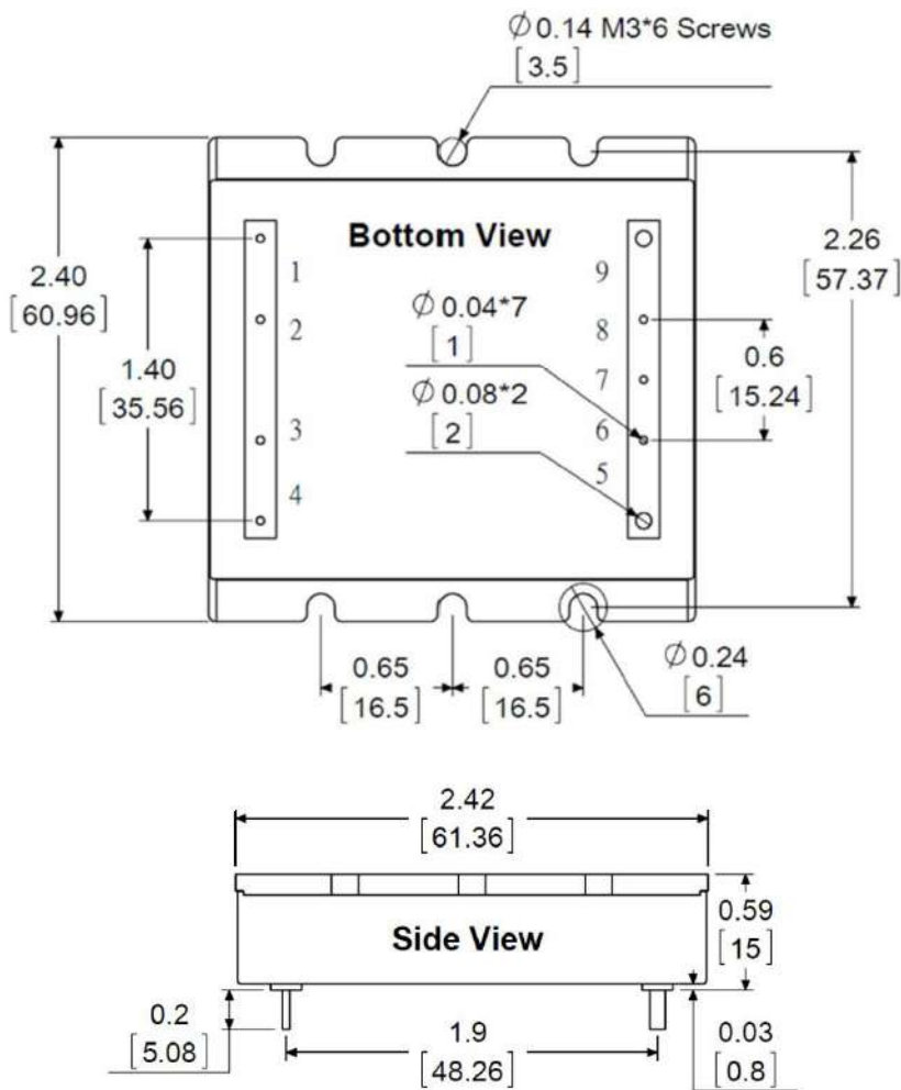
尺寸图-B (金属壳法兰片)
